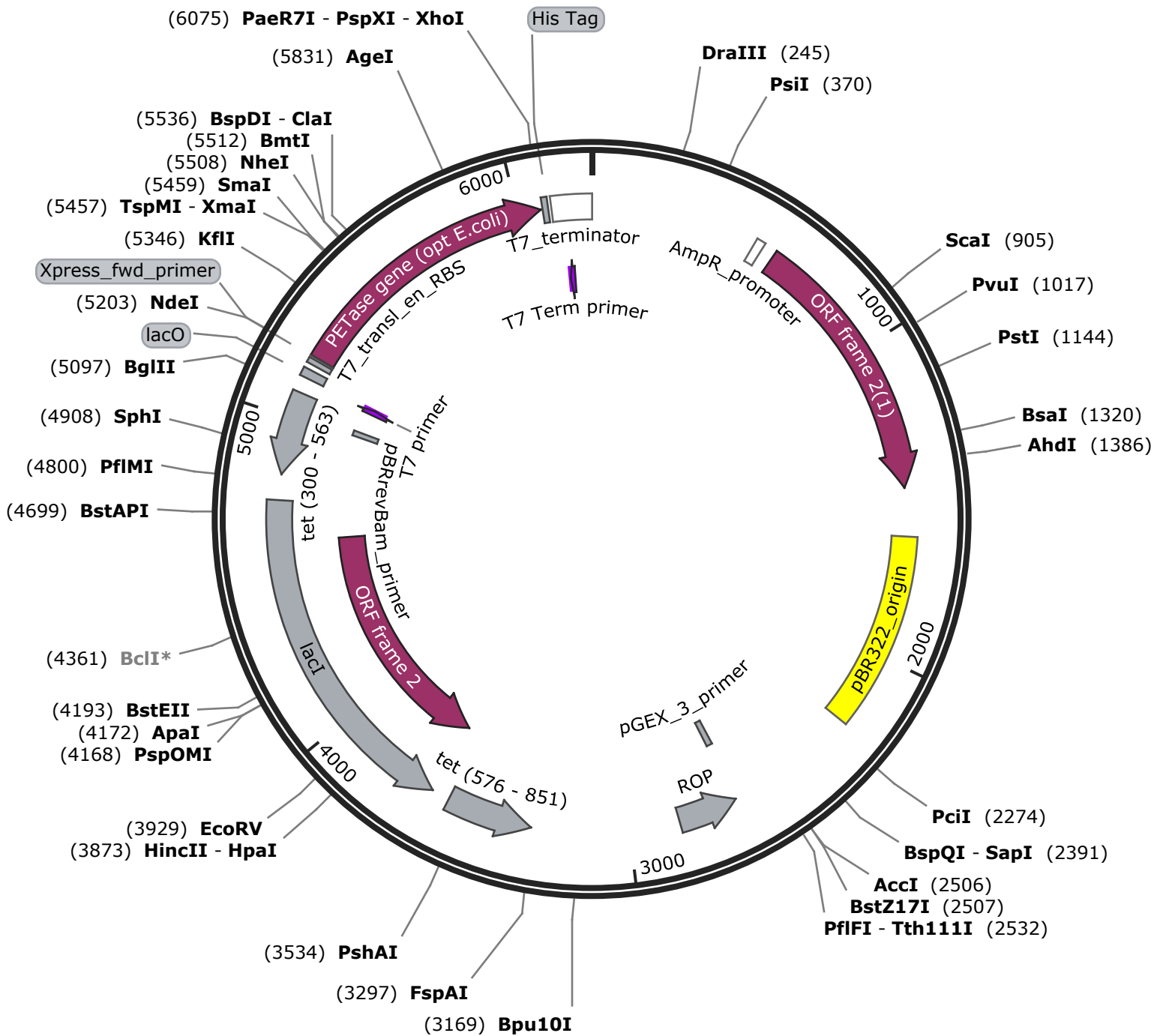
pCJ135 Ideonella sakaiensis PETase gene in pET-21b(+)
