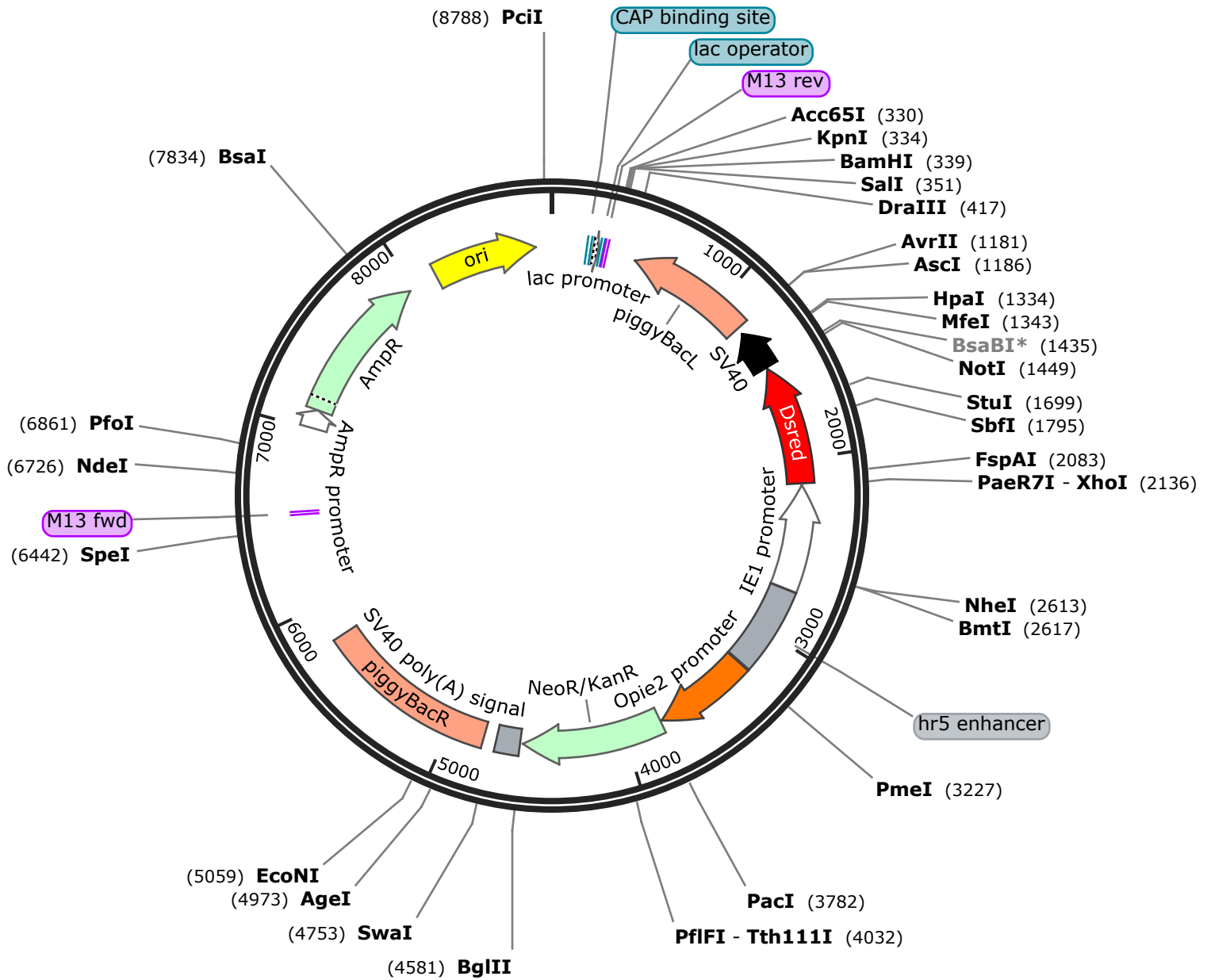
Opie2-NeoR=pBac-HR5Ie1-dsRed+Opie2-NeoR 8826 bp
