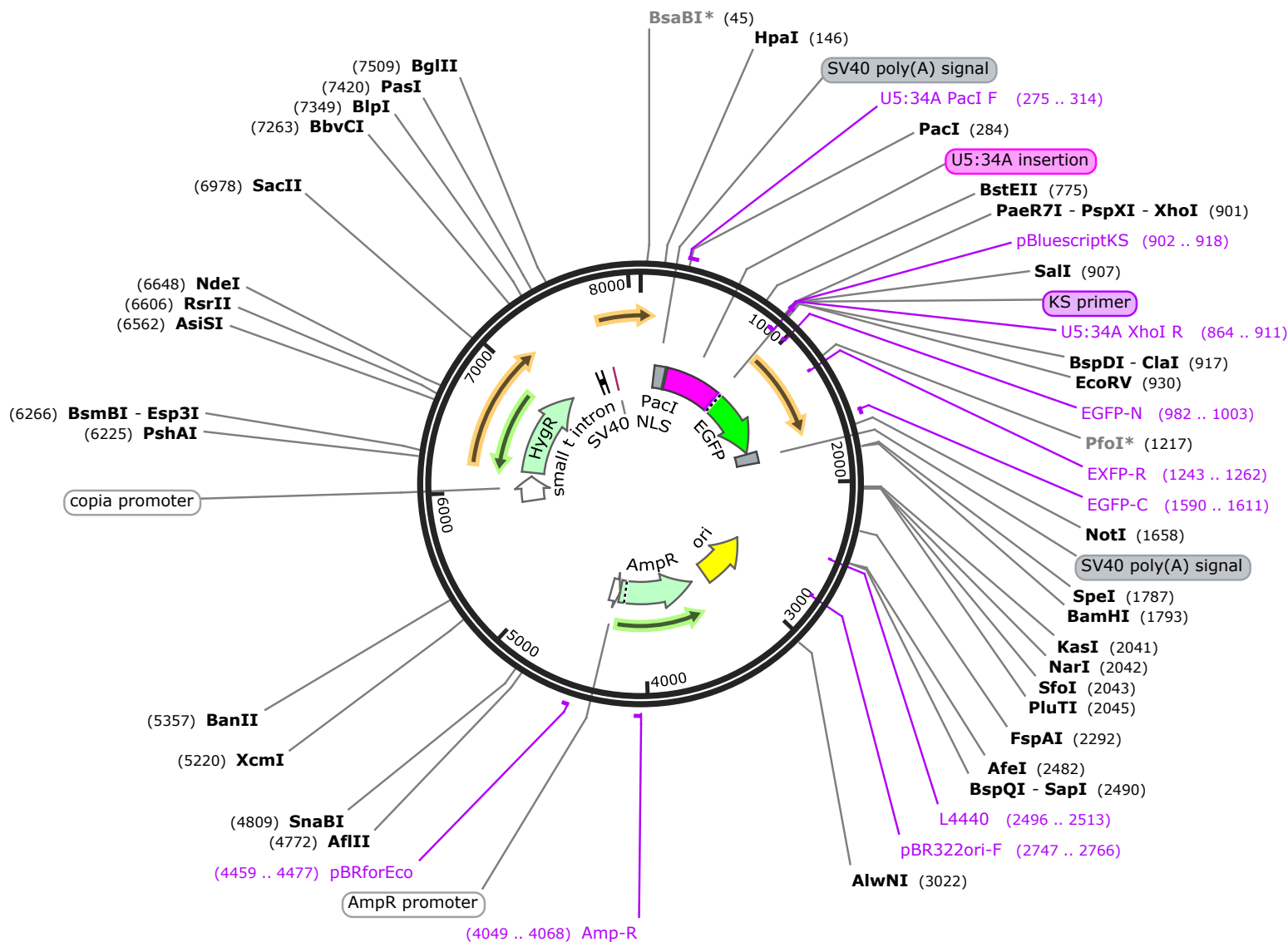
Hy_U5 34A eGFP SV40 8079 bp
