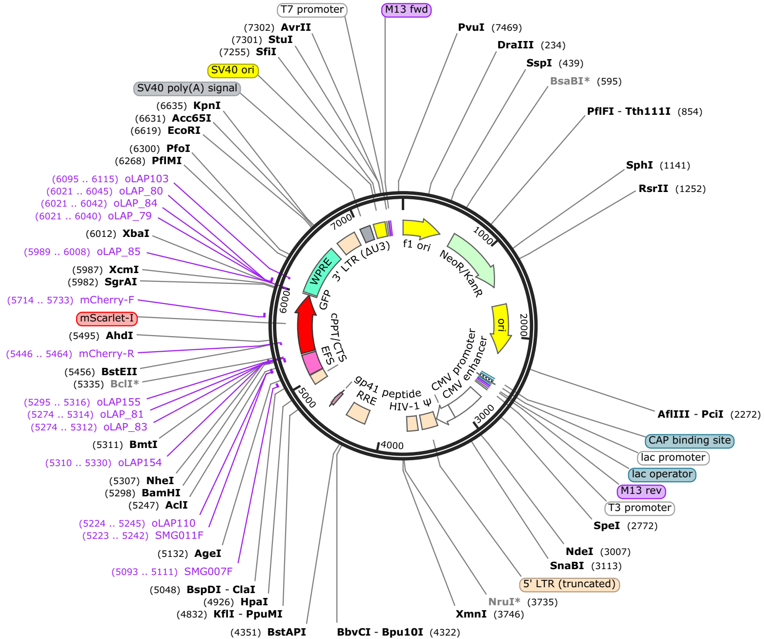
pLP202_pCCL_EFSp_Soluble mScarletI_WPRE(UTR)
