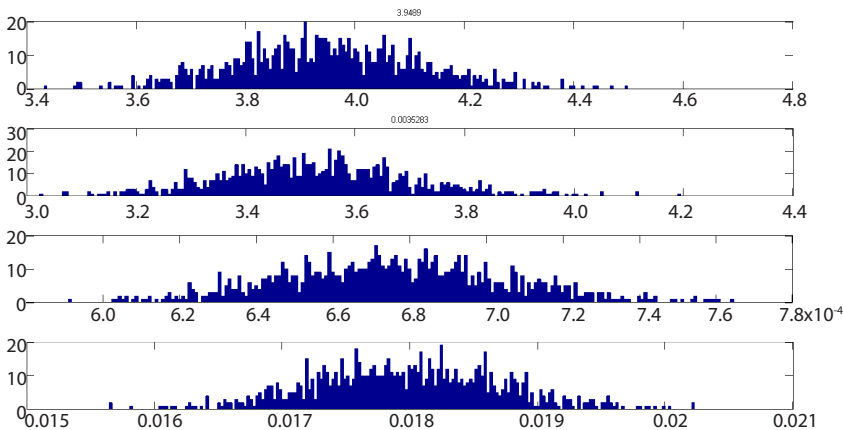
mKO2 total protein parameter distributions
