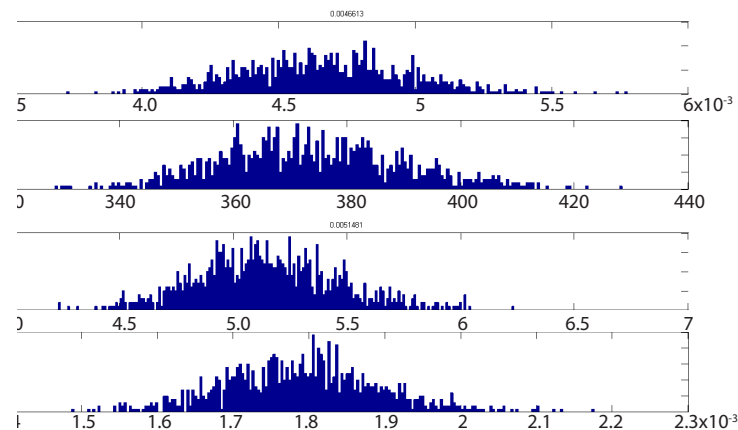
mKO2 mature protein parameter distributions
