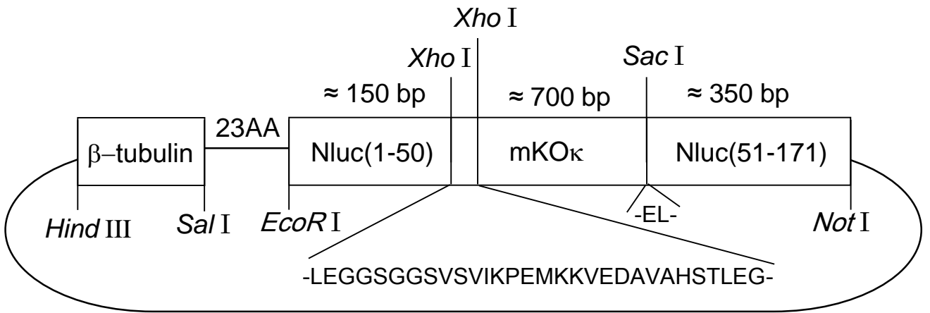
pcDNA3-tubulin-OeNL
