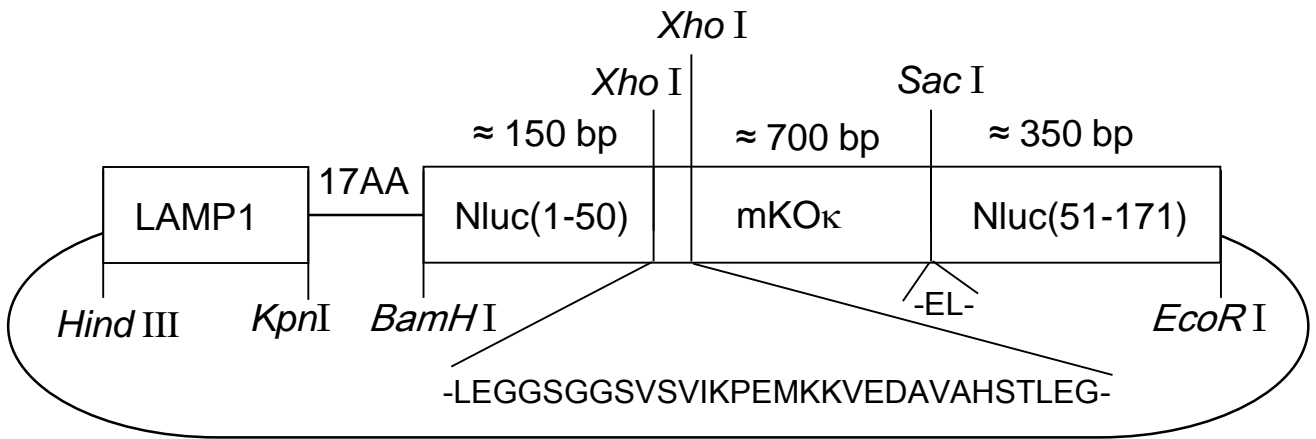
pcDNA3-LAMP-OeNL
