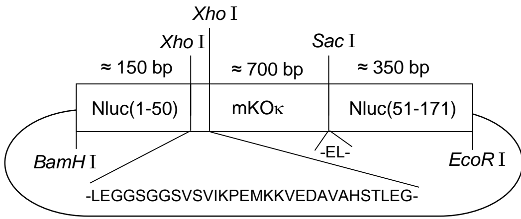
pRSETb-OeNL
